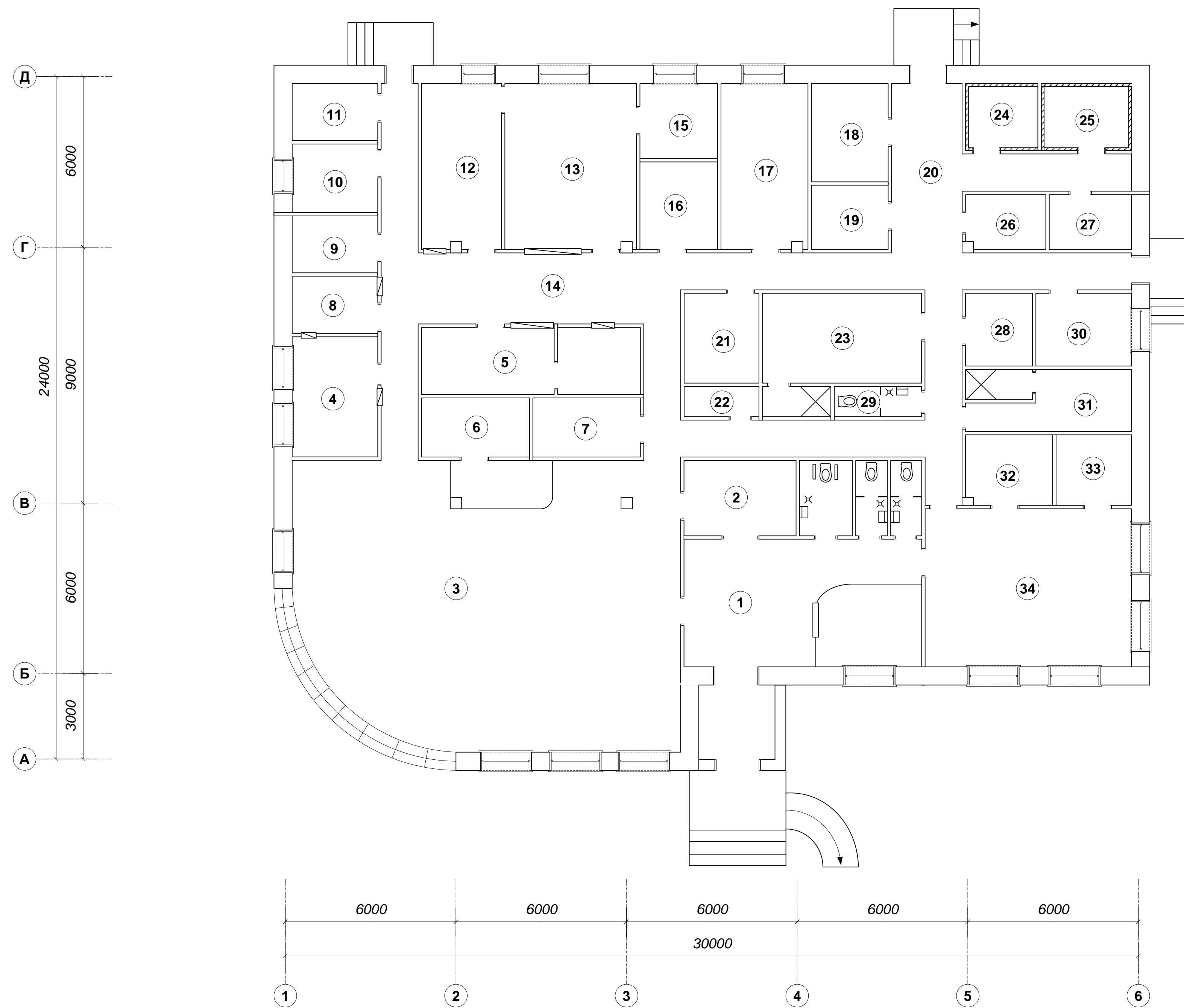
План на отметке ±0,000
