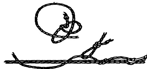
Петля на двойной хребтине
