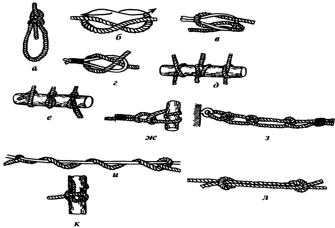
Морские, применяемые аквалангистами: а - беседочный; б - прямой; в - рифовый; г - шкотовый; д - выбленочный; е - удавка; ж - простой штык; з - штык со шлагом; и - стопорный; к - шлюпочный; л - связывание чужими концами
