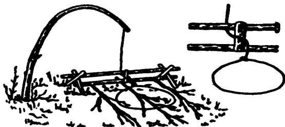
Пружок на рябчика
