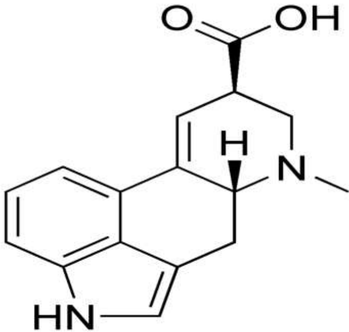
Лизергиновая кислота
