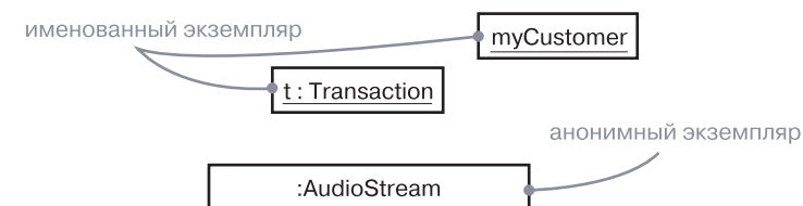
Рис. 13.2. Именованные и анонимные экземпляры
