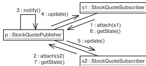
Рис. 16.7. Организация потока управления
