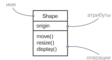
Рис. 4.1. Классы
