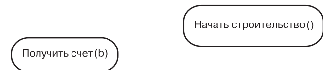
Рис. 20.3. Узлы деятельности
