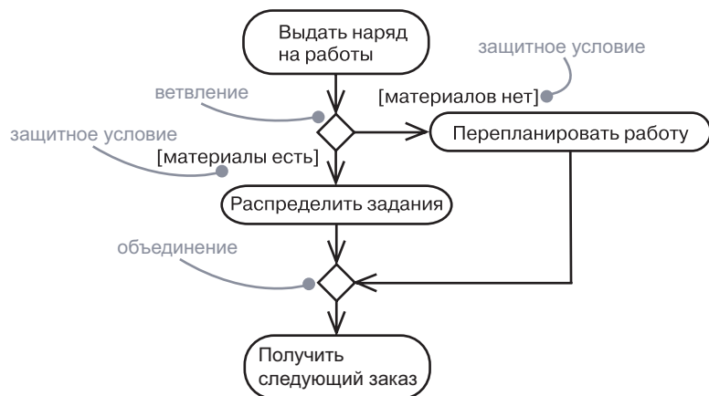
Рис. 20.5. Ветвление
