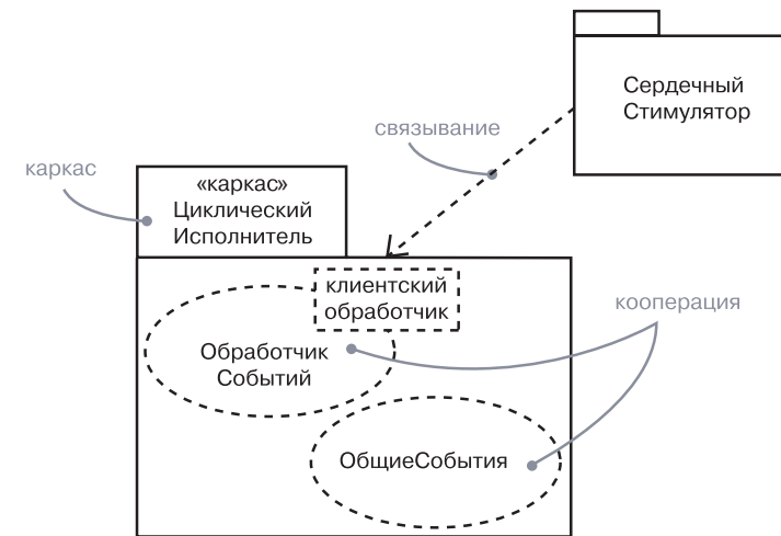
Рис. 29.3. Каркасы
