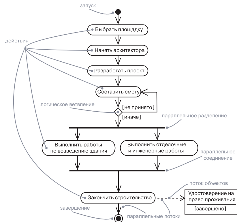
Рис. 20.1. Диаграмма деятельности
