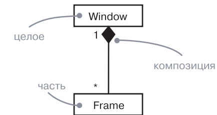
Рис. 10.6. Композиция
