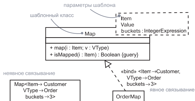
Рис. 9.7. Шаблонные классы
