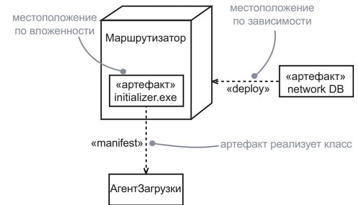
Рис. 24.3. Местоположение
