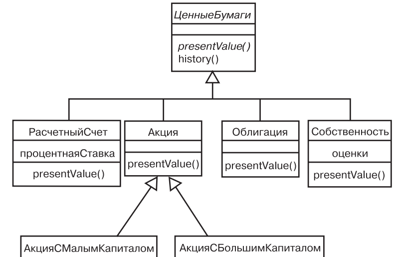
Рис. 5.10. Связи наследования
