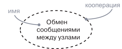
Рис. 28.1. Кооперации
