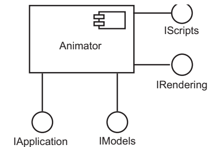
Рис. 15.7. Моделирование AP
