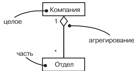
Рис. 5.7. Агрегация
