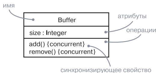
Рис. 23.3. Синхронизация
