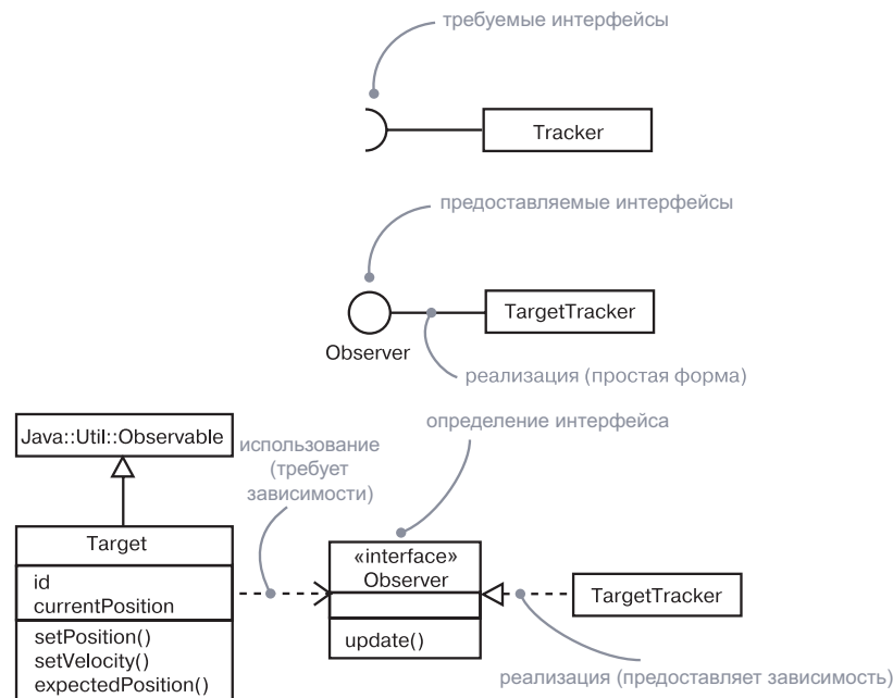
Рис. 11.4. Реализация
