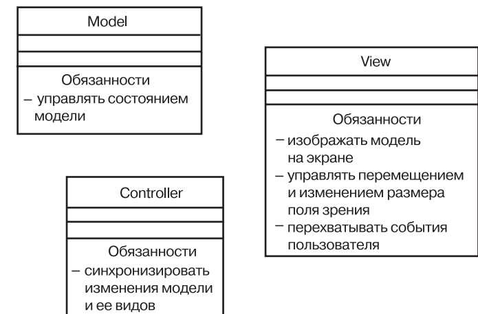
Рис. 4.10. Моделирование распределения обязанностей в системе
