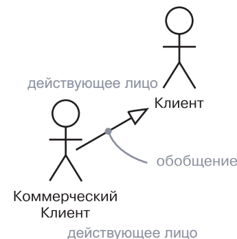
Рис. 17.3. Действующие лица
