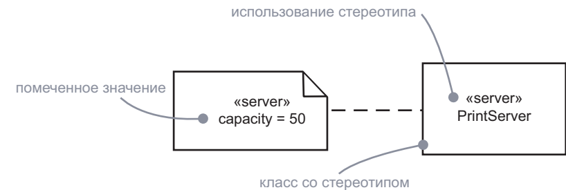
Рис. 6.7. Помеченные значения
