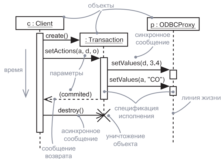
Рис. 19.2. Диаграмма последовательности
