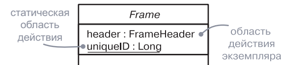
Рис. 9.4. Область действия
