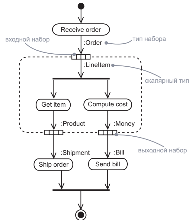
Рис. 20.9. Область расширения
