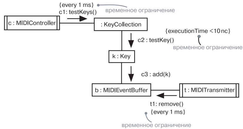
Рис. 24.2. Время
