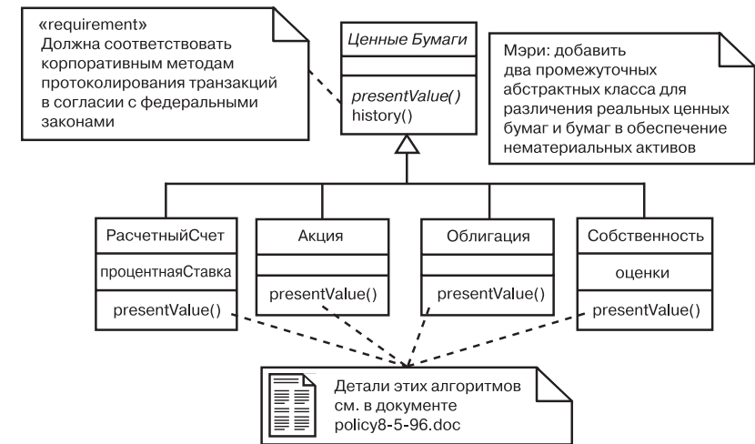
Рис. 6.9. Моделирование комментариев
