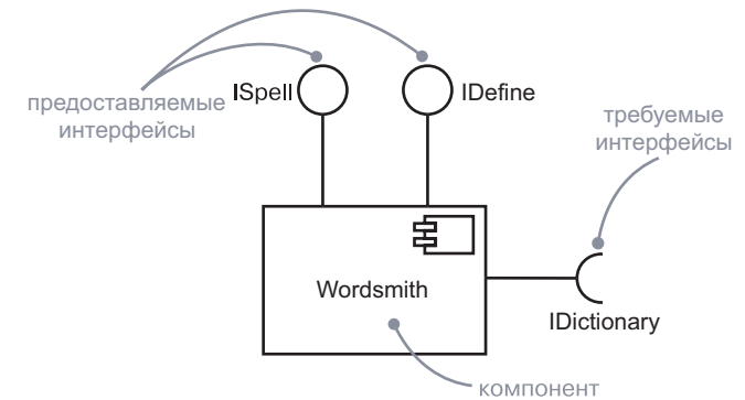
Рис. 11.1. Интерфейсы
