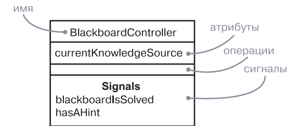
Рис. 23.1. Активный класс
