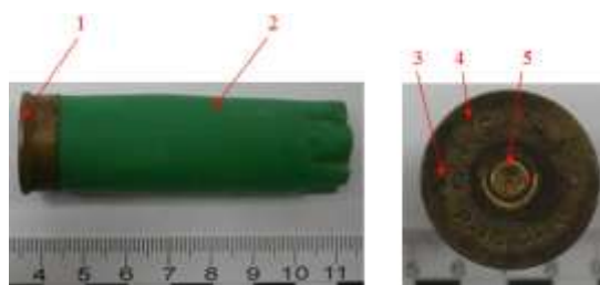
Рис. 6. Вид цилиндрической части и шляпки гильзы
