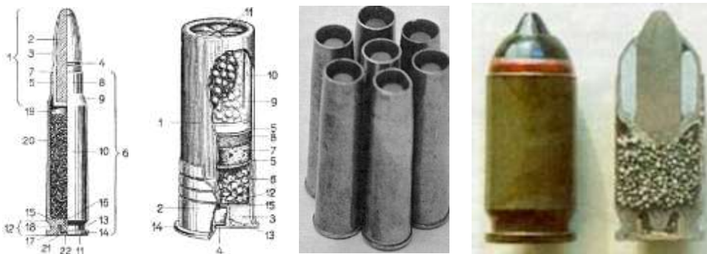
Рис. 1. Патроны к нарезному и гладкоствольному оружию, револьверу "Наган" и ПМ
