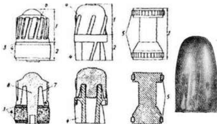
а) кончик головки б) головная ( оживальная ) часть в) ведущая (цилиндрическая) часть; г) донная часть ( донце ) пули. Рис. 3. Снаряды к патронам гладкоствольных ружей и нарезному оружию
