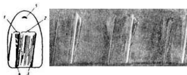
Рис. 4. Следы на пуле и развертка нарезов на пуле
